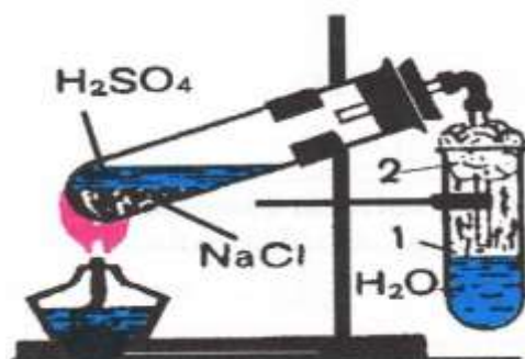
Şəkil 1. Laboratoriyada xlorid turşusunun alınması.
