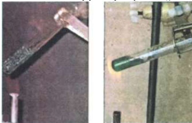
Şəkil 4. Mayelərin sınaq şüşəsində qızdırılması: a – sınaq şüşəsində tutqaca bərkidilmiş vəziyyətdə; b – sınaq şüşəsində ştativin pəncəsinə bərkidilmiş vəziyyətdə.
