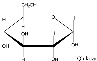
Qlükoza
