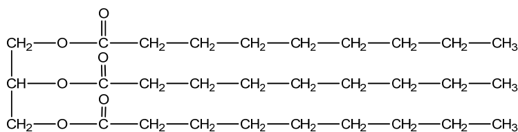
Triqliserid
