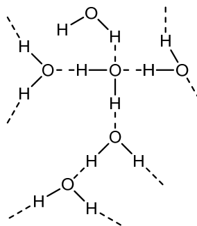
Şəkil 1. Su molekulları arasında hidrogen rabitəsi.
