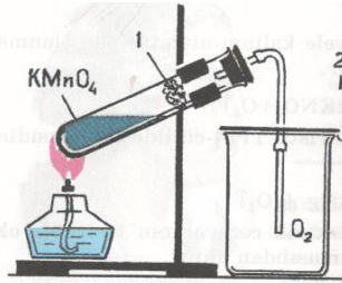
Şəkil 2. Havanı sıxışdırıb çıxarmaqla oksigenin yığılması: 1- şüşə pambıq; 2 – hava;
