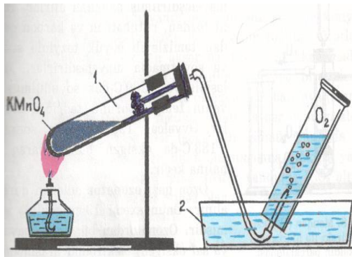
Şəkil 1. Suyu sıxışdırıb çıxarmaqla oksigenin yığılması: 1 – şüşə pambıq; 2 – su
