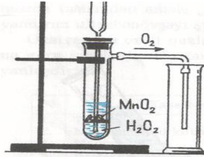
Şəkil 3. Manqan (IV) oksidin iştirakı ilə hidrogen-peroksidin parçalanması reaksiyasının sürətlənməsi.
