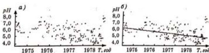
Şəkil 1. Yağış suyunun pH dəyərini dəyişdirməsi probleminin müzakirəsi: a-statik məlumatların işlənməsindən əvvəl; b-statik məlumatların işlənməsindən sonra.
