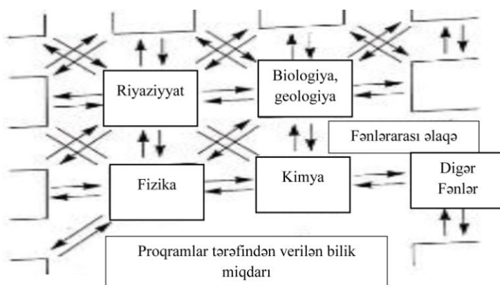
Sxem 3. Kimya akademik fənlər sisteminin bir elementi kimi
