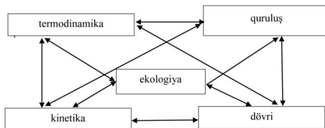
Sxem 5. 5 bloktan ibarət sistemə kursun qurulması
