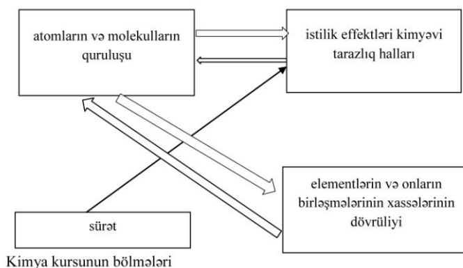
Sxem 2. Kimya kursunun əhəmiyyətli quruluşu atomların və molekulların quruluşu, kimyəvi rabitələr və molekullararası qarşılıqlı təsir.
