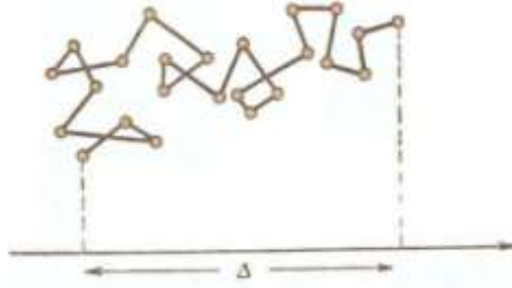
Şəkil. Hissəciyin Broun hərəkətinin sxemi.
