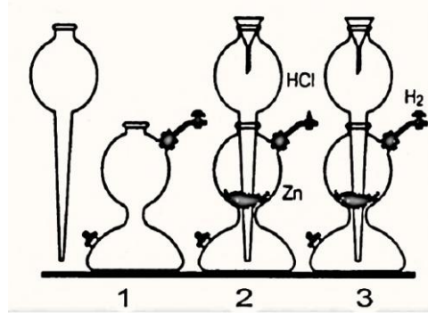
Kipp aparatında Hidrogenin alınması
