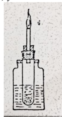
Sadə Kipp aparatı
