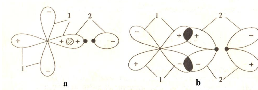
Şəkil 1. Keçid metalın CO liqandı ilə dativ rəbitəsi
