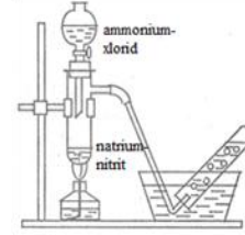
Şəkil 6. Azotun ammonium- nitritdən alınması
