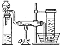
Şəkil 3. Azotun maye havadan alınması
