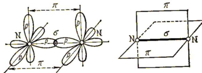
Şəkil 2. Azot molekulunda \sigma - və \pi -rabitələrin əmələ gəlməsi
