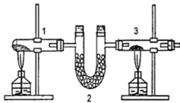
Şəkil 9. Azotun maqneziumla qarşılıqlı təsiri
