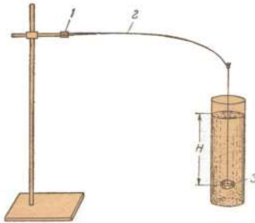
Şəkil 1. Fiqurovski sedimentometri:
