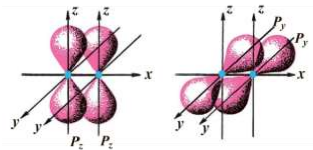
Şəkil 2. \pi -rabitənin yaranması
