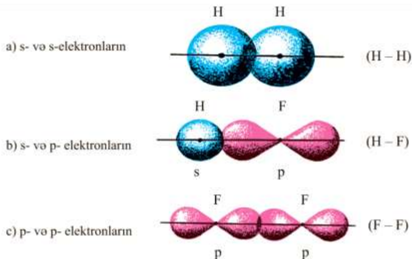
Şəkil 1. Rabitənin əmələ gəlməsi zamanı elektron buludlarının örtülmə sxemi
